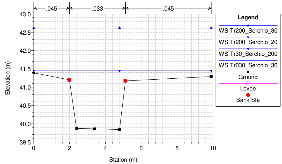
Fosso Carraia - Progetto Definitivo 2006 Plan: Carraia aggiornato 1 6/21/2021
